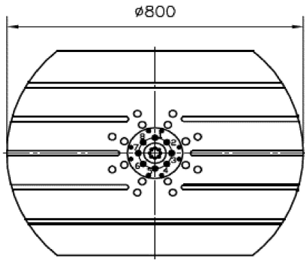
U-800工作台尺寸
