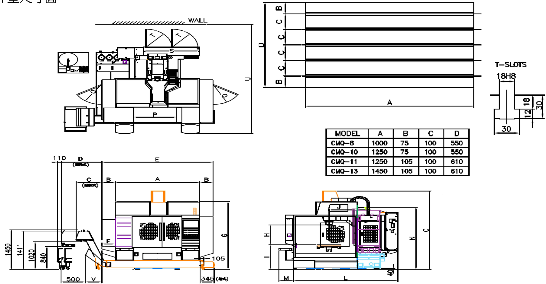
CMQ-8外型尺寸圖
