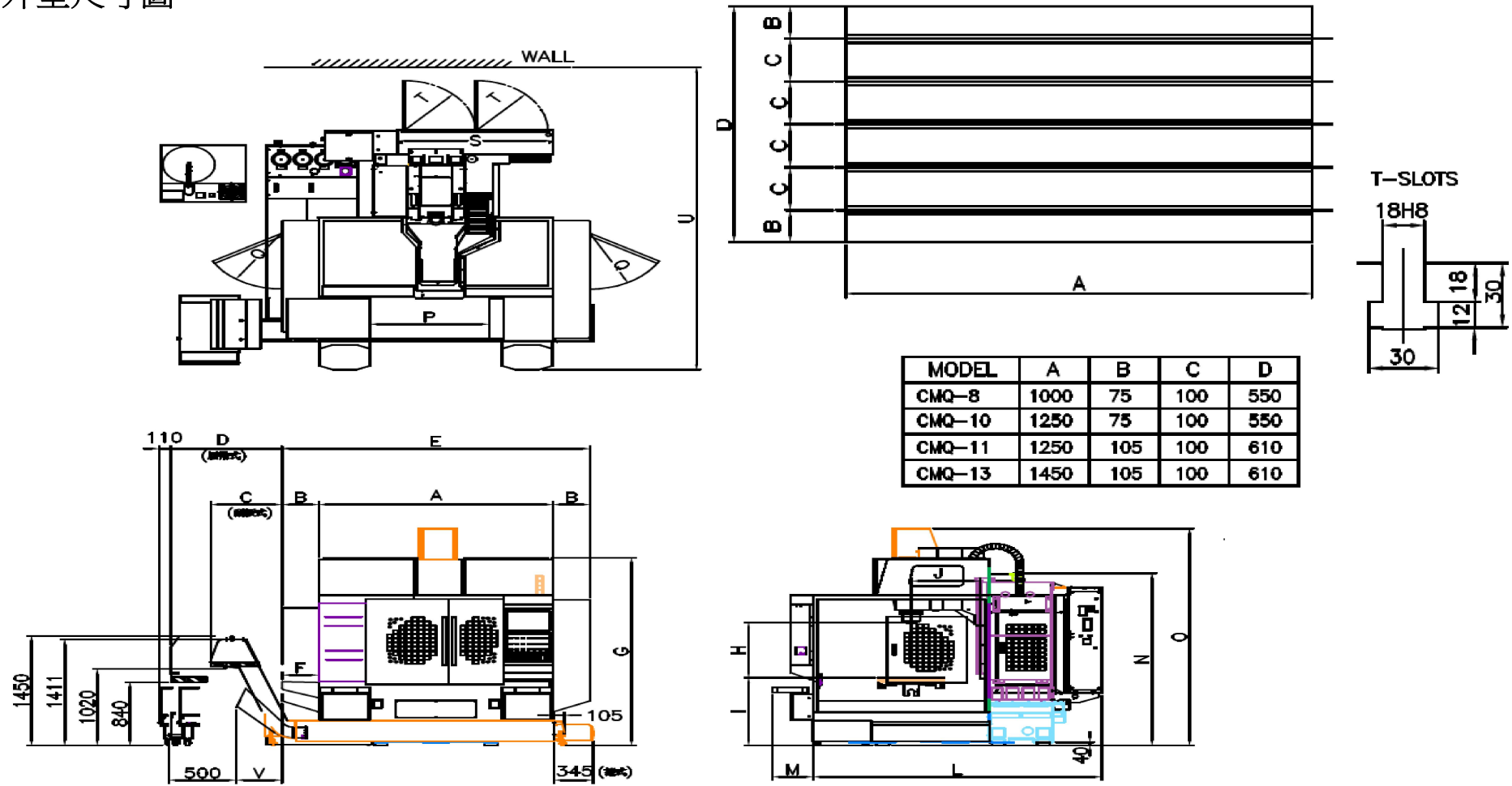
CMQ-13外型尺寸圖
