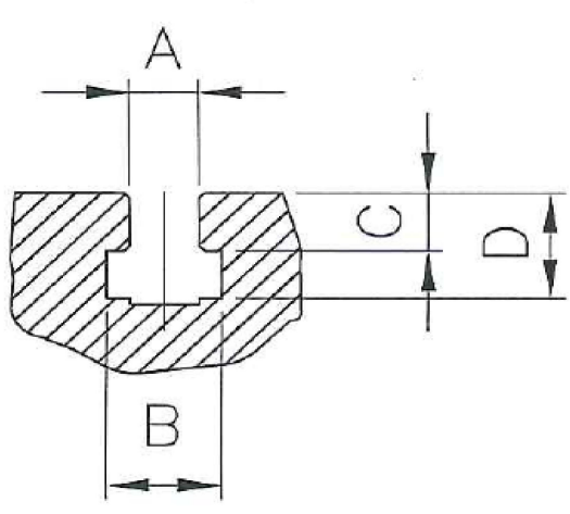
T型溝詳圖
